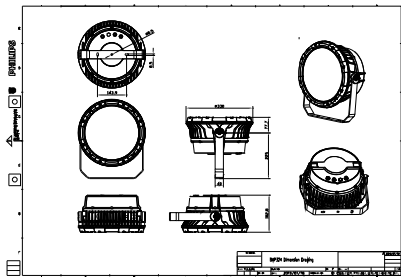
BVP324 72LED RGBNW 220V 15 DMX D2
