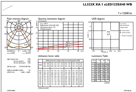
IFGU1_LL523XXA1xLED123S840WB
